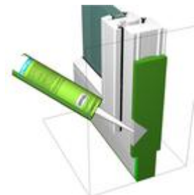
Bild 2: Spritzklotz einfüllen
